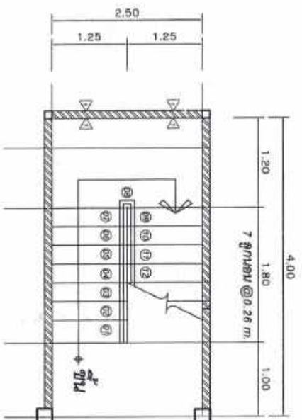
แบบขยายแปลนบันไดชั้นล่าง
