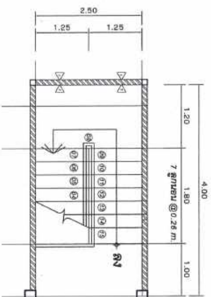
แบบขยายแปลนบันไดชั้นบน
